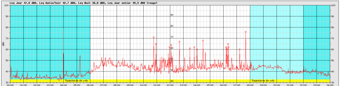
Figure 3 : Mouans-Sartoux le 25/01 : record de 16 survols
